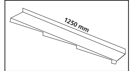
Veggbeslag (høyre/venstre)
